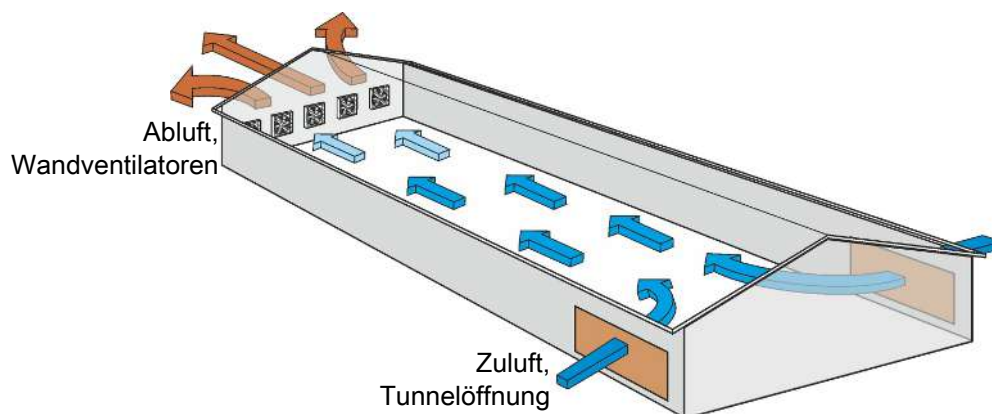
Abb. 1: Prinzip der Tunnellüftung
