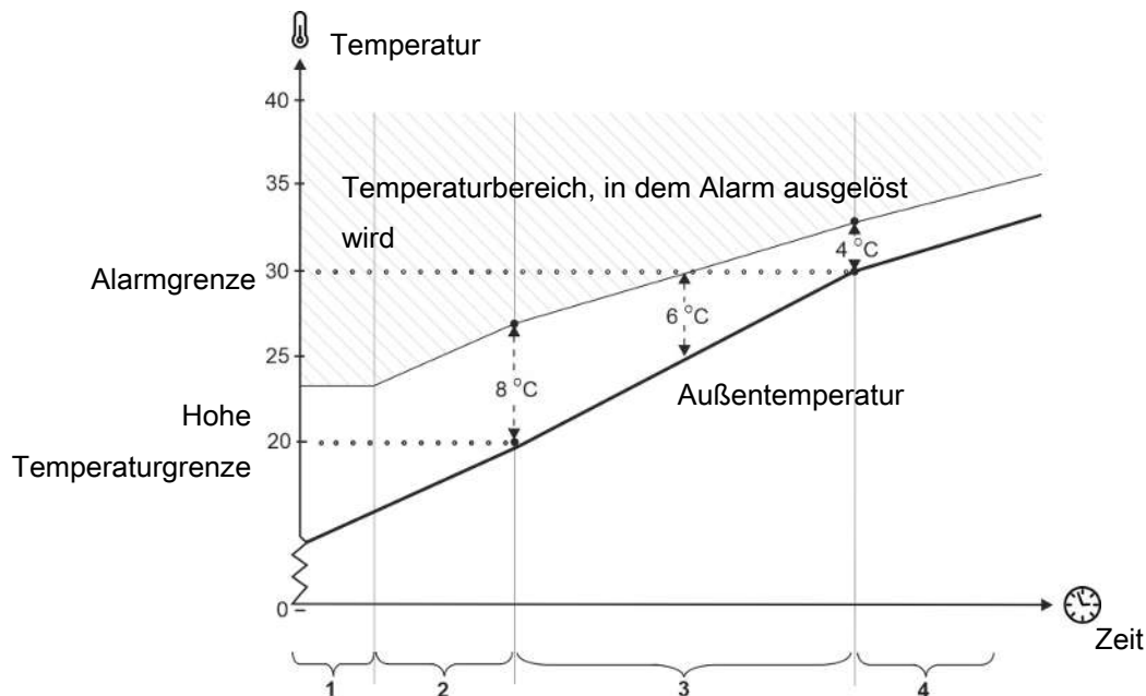
Abb. 11: Sommertemperatur bei 20°C und 30°C Außentemp.
