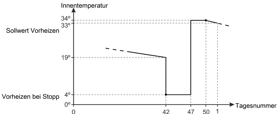
Abb. 10: Beispiel für Einstellung der Funktion Vorheizen
