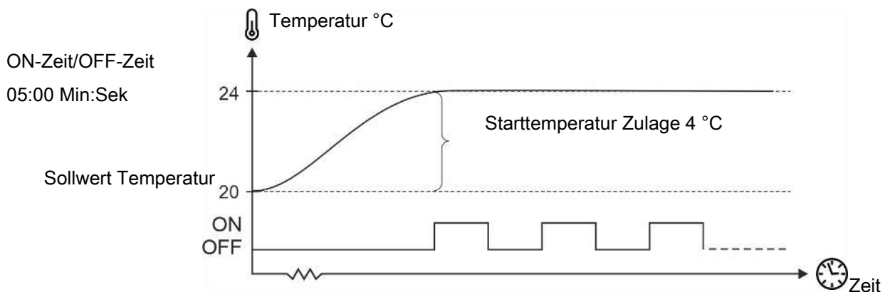
Abb. 3: Relaisgesteuerter Umluftventilator (EIN/AUS) basierend auf der Temperatur
