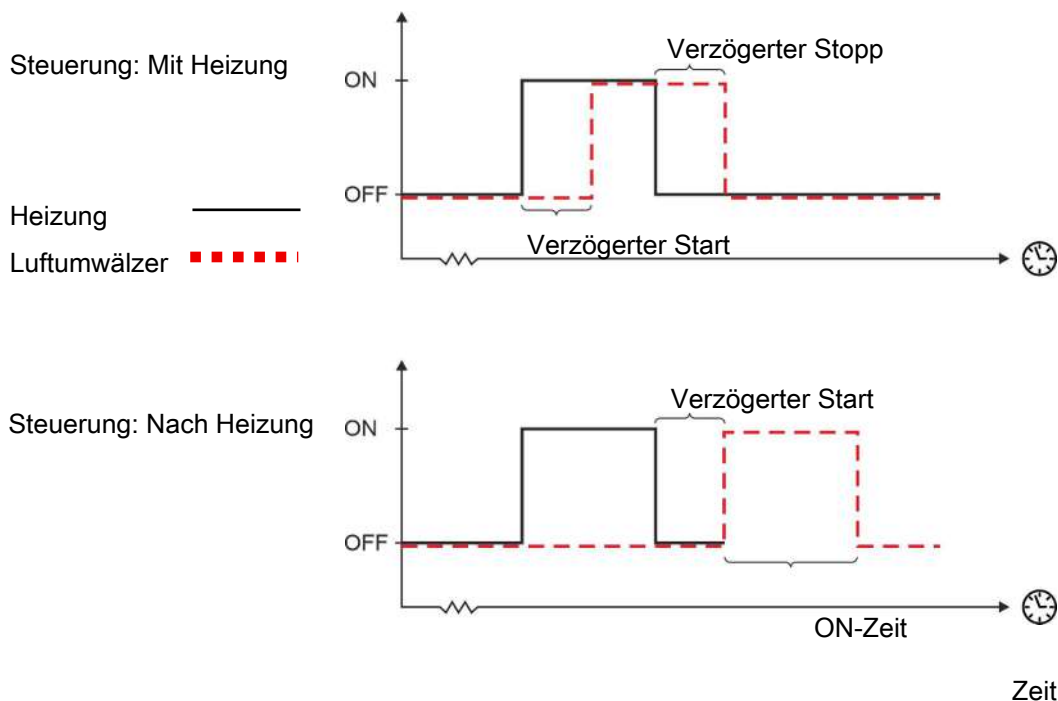
Abb. 6: Steuerung durch Heizquelle
