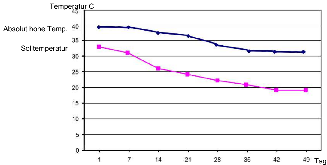
Abb. 12: Beispiel Absolut hohe Temperatur Alarm.
