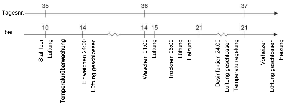
Abb. 9: Verlauf der Pausenfunktionen
