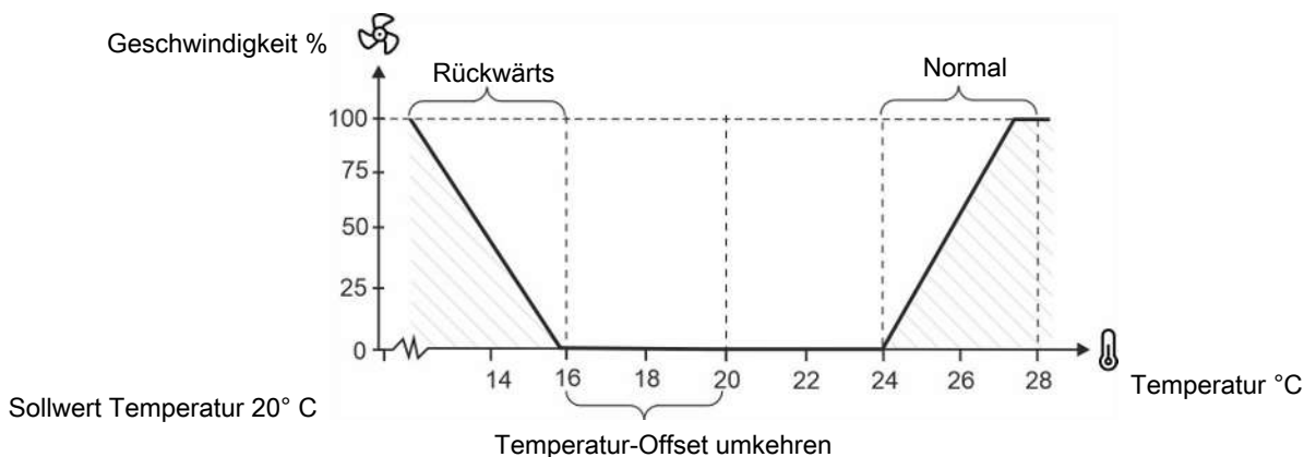
Abb. 5: 0–10 V-geregelter Luftumwalzer mit Umschaltrelais
