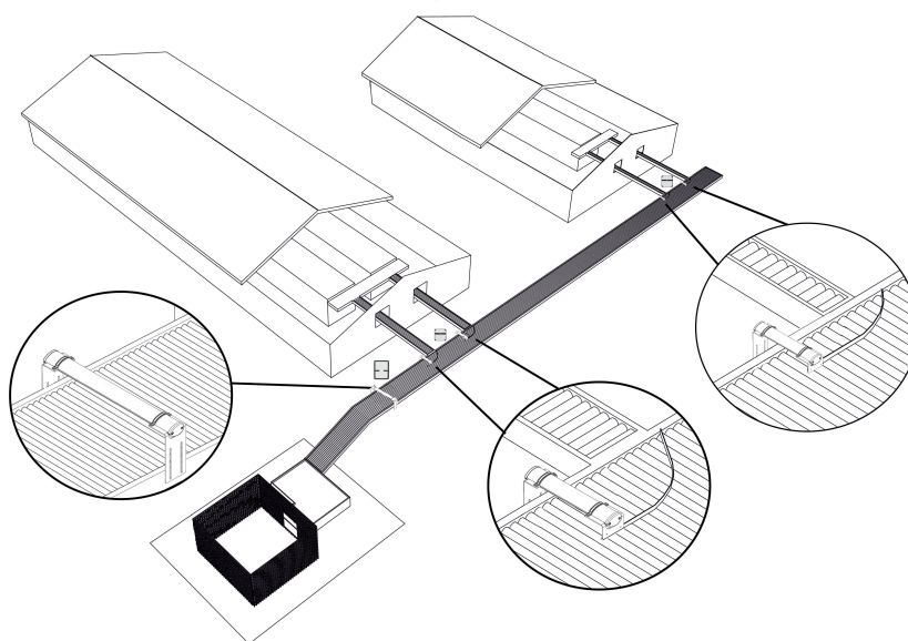
Abb. 16: Schematische Darstellung für die Positionierung von automatischen Eierzählern.
