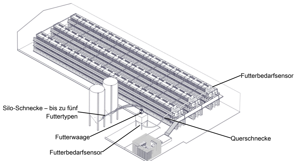
Abb. 6: Schematische Darstellung der Ausfütterung an Legehennen für Käfighaltung.
